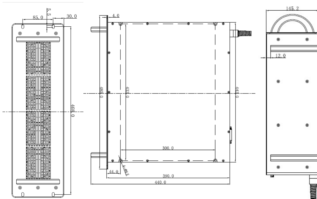
100W 尺寸图
